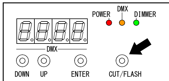
Sai-500CBコントロールパネル
